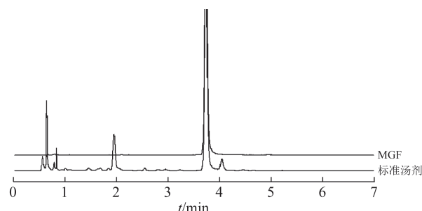
图1 知母标准汤剂的 MGF 含量测定的 UPLC-PDA 图
