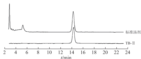
图2 知母标准汤剂的TB-Ⅱ含量测定的UPLC-ELSD图
